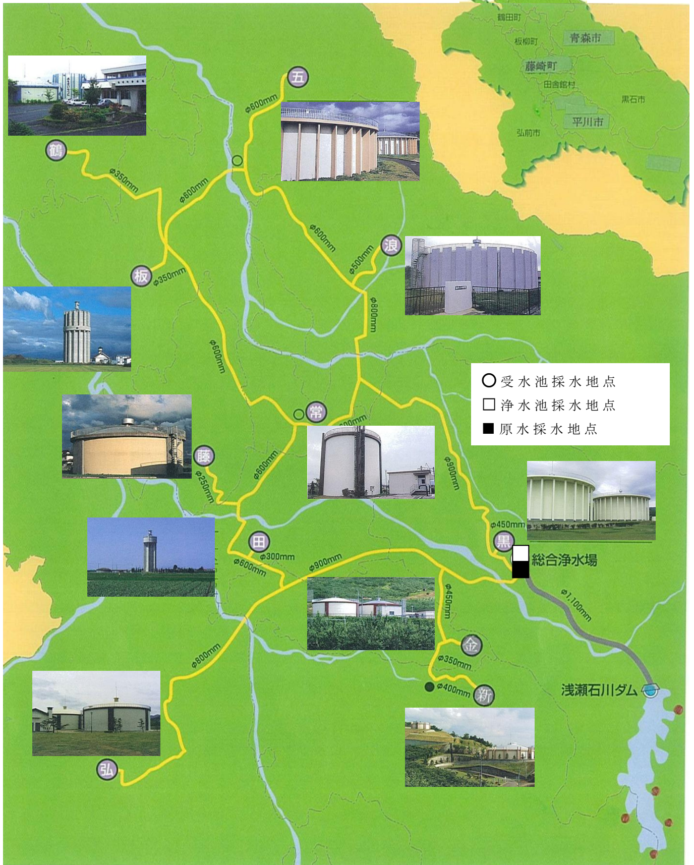
図：送水系統及び採水地点図
